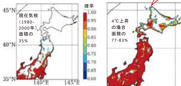
図17 竹林の生育に適した環境と予測された地域 出典15より
