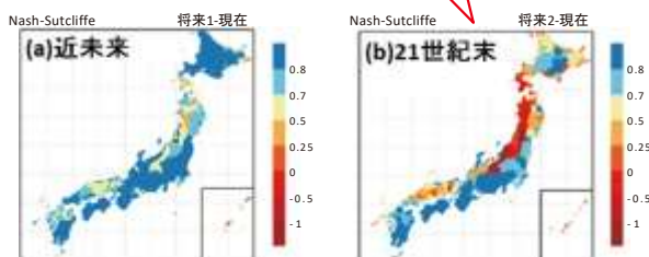
図20 気候変動に伴う日本各地の河川流況の将来変化 出典18より一部改変
